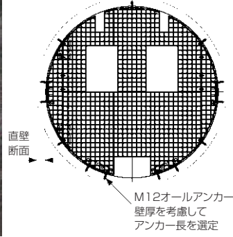
アンカー仕様例
