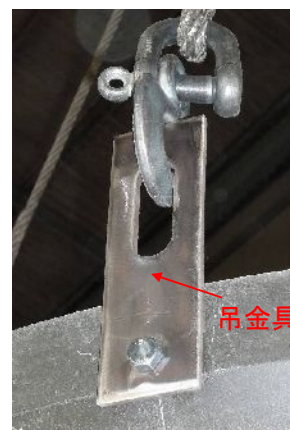
0~3号用吊金具
