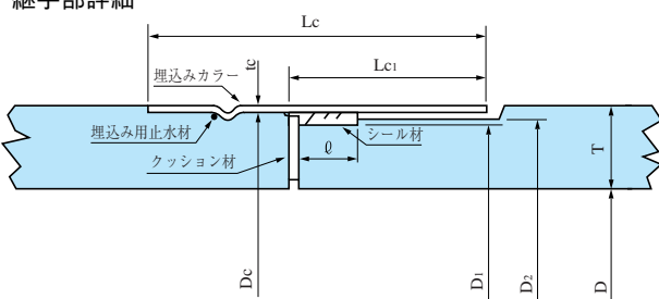
継手部詳細
