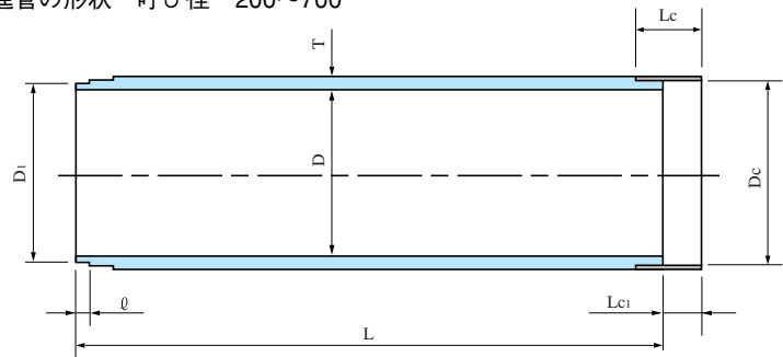
推進管の形状 呼び径 200～700
